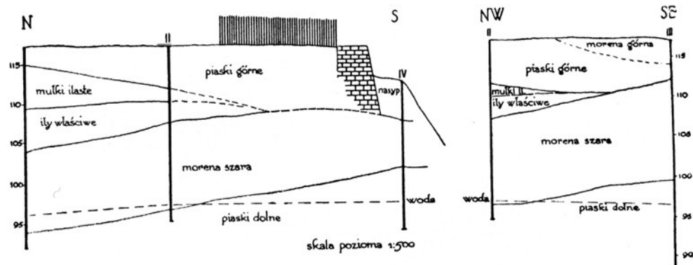
PRZEKROJE SCHEMATYCZNE DO PLANU (NA STR. 35) — W OPRACOWANIU DRA BR. HALICKIEGO. CYFRAMI RZYMSKIMI OZNACZONE SĄ OTWORY WIERCEŃ GRUNTU.
