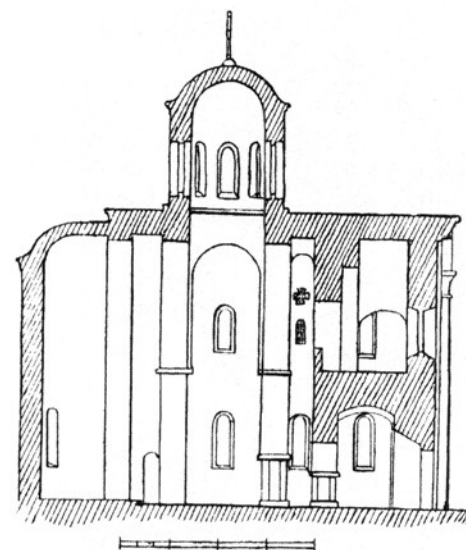
CERKIEW ZBAWICIELA I ŚW. EUFROZYNY W POŁOCKU (POL. XII W.). PRZEKRÓJ PODŁUŻNY.
